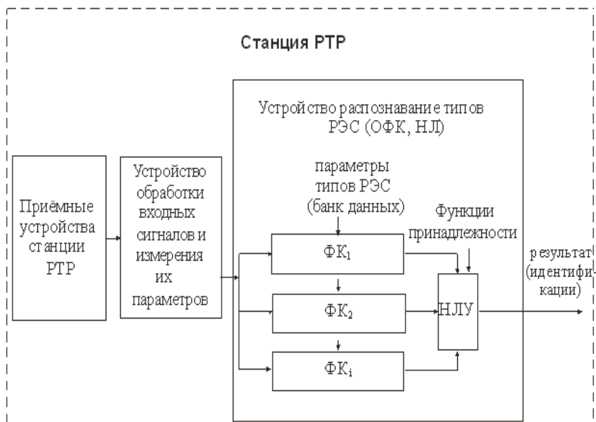
Рис. 1. Структурная схема станции радиотехнической разведки с устройством распознавания типов, использующего комплексирование методов ОФК и НЛ
