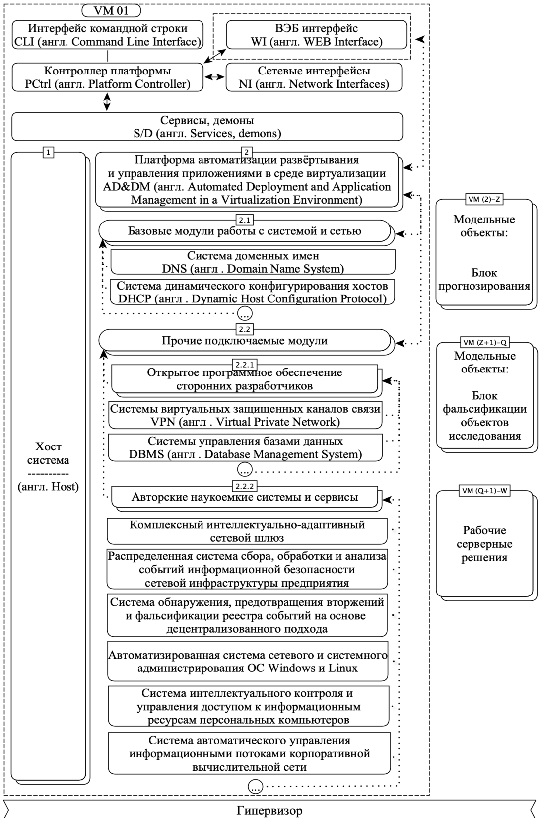
Рис. 3. Архитектура системы интеллектуально-адаптивного управления сетевой инфраструктурой предприятия
