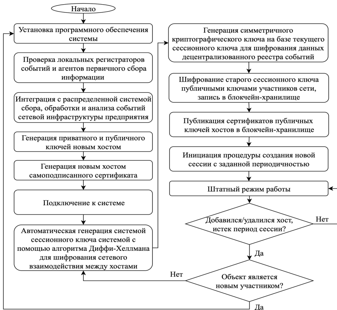
Рис. 1. Блок-схема предлагаемого метода: подключение к системе, инициализация сетевого взаимодействия
